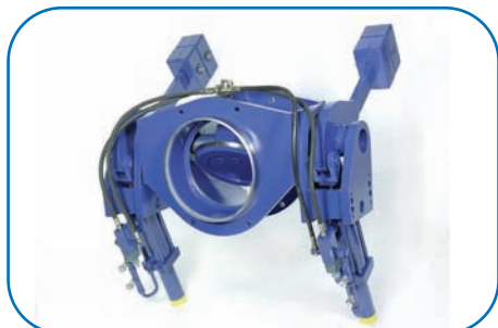
510 型旋启式止回阀 DN 400 焊接连接，双侧都配有杠杆和重块， 带有油制动器，对付较高的回流压力
